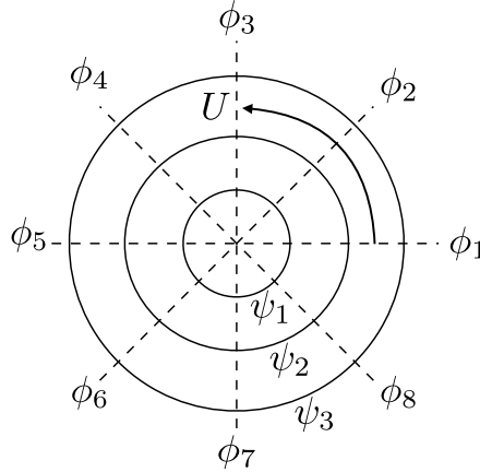
FIGURE 8.2 – Tourbillon. Lignes de courant et équipotentiellles.
