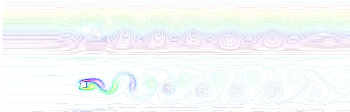
FIGURE 2.5 – Écoulement instationnaire dans le sillage d'un obstacle de section carrée, résultat de simulation numérique. En haut, lignes de courant. En bas, lignes d'égaux valeur de la vortacité au même instant.
